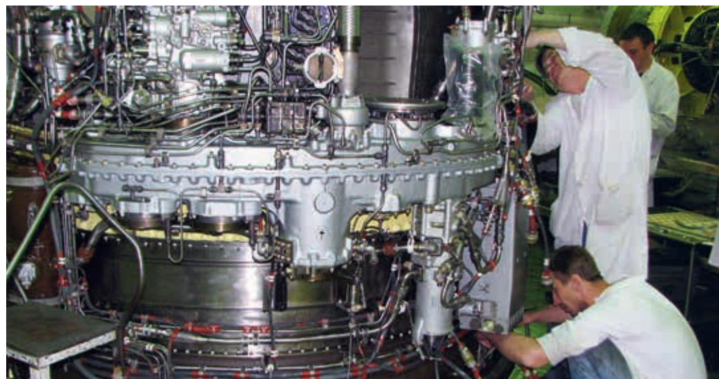
Сборка двигателя ПС-90А
